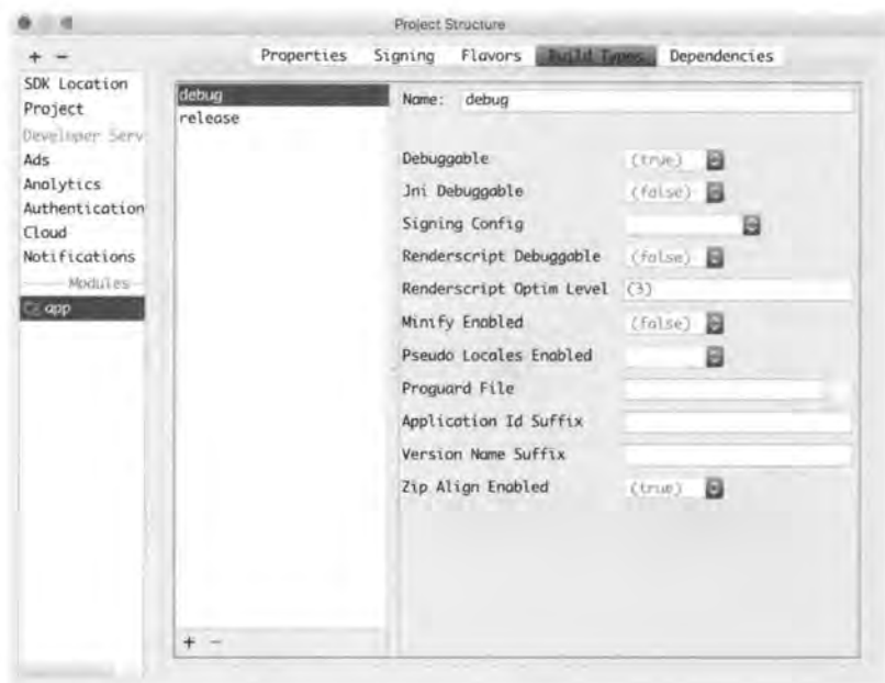
图 4.52 Project Structure 的构建版本
