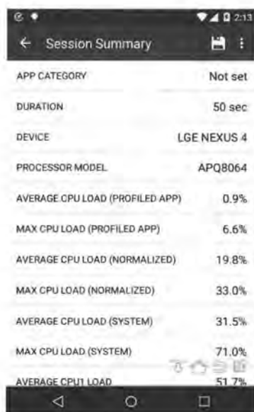
图 6.110 App Tune-up Kit 详细数据
