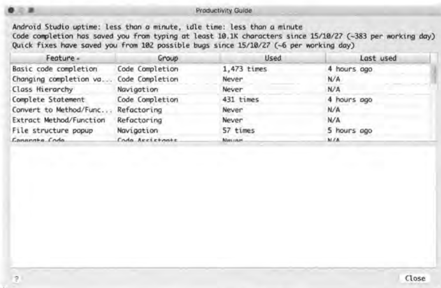
图 3.110 Productivity Guide 信息
