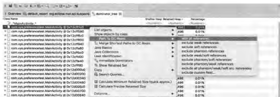
图 6.77 Path To GC Roots
