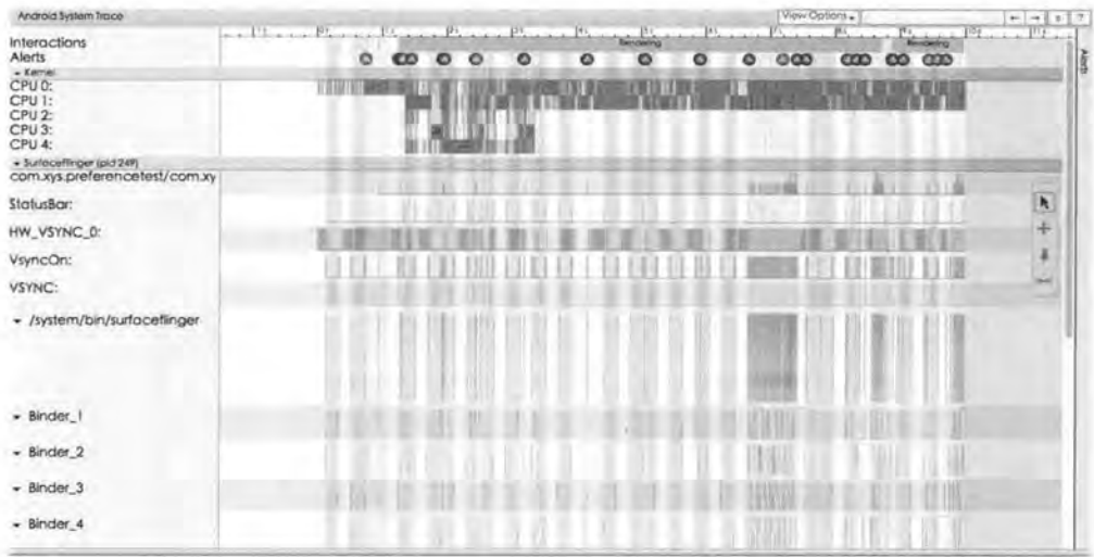
图 6.25 r23 版本 Systrace 数据结果图
