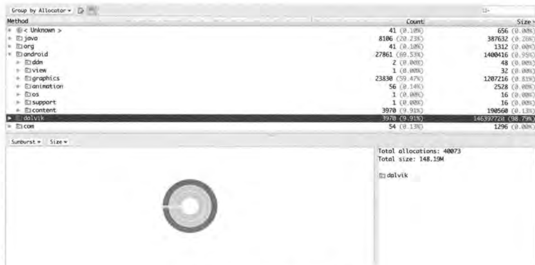
图 6.57 Allocation Trackinging 数据
