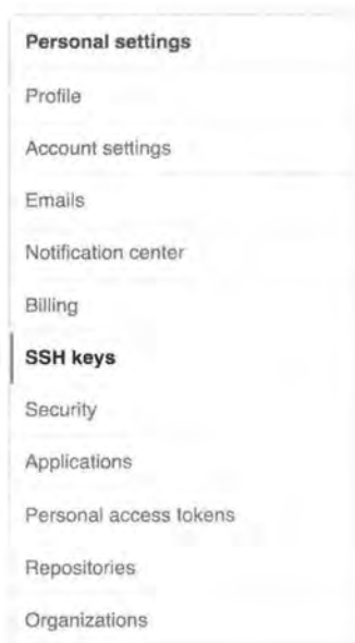
图 2.8 Github Setting
