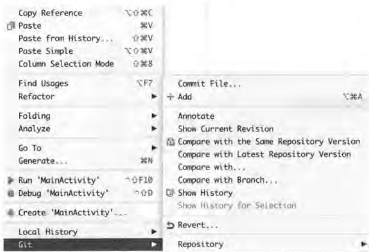
图 3.91 Git 操作
