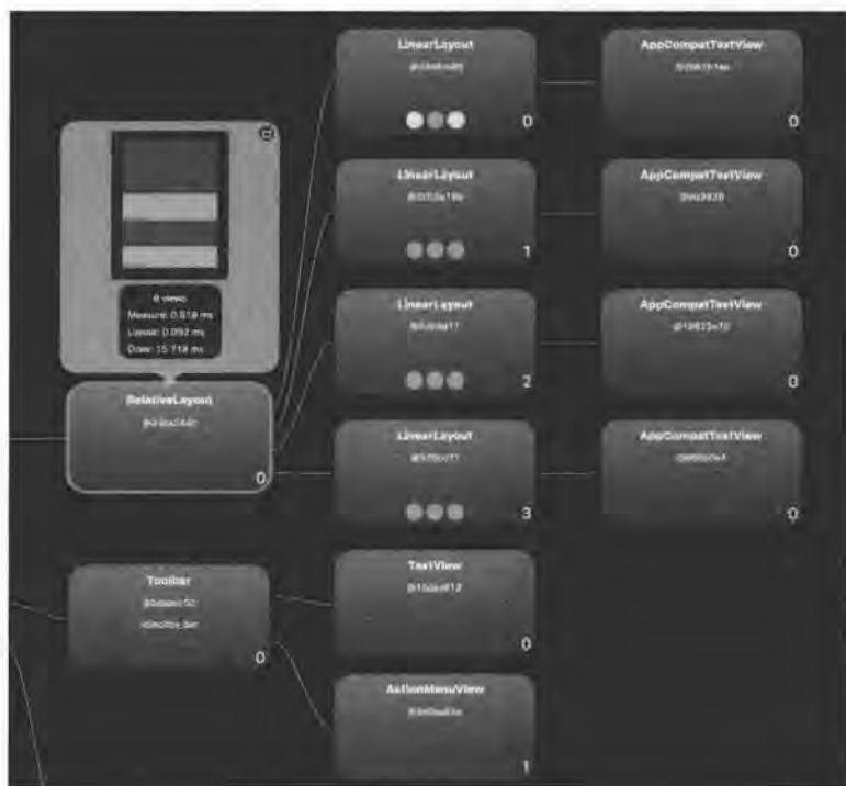
图 6.6 Hierarchy Viewer
