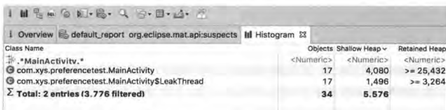
图 6.70 过滤条件
