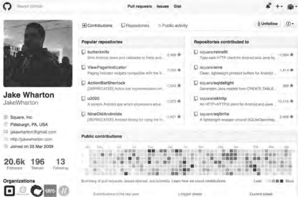
图 7.5 Github
