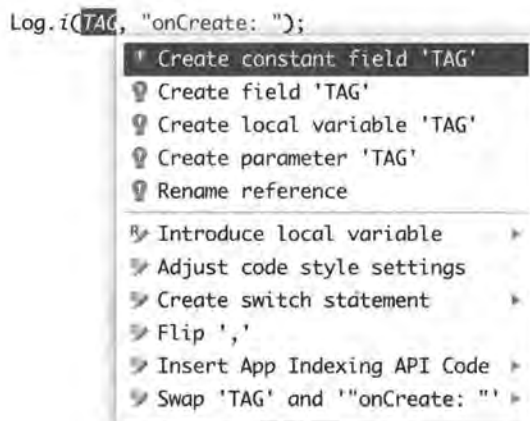
图 3.33 快速修复
