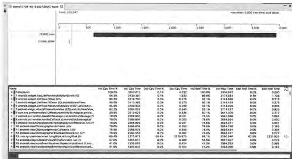
图 6.39 Traceview 数据
