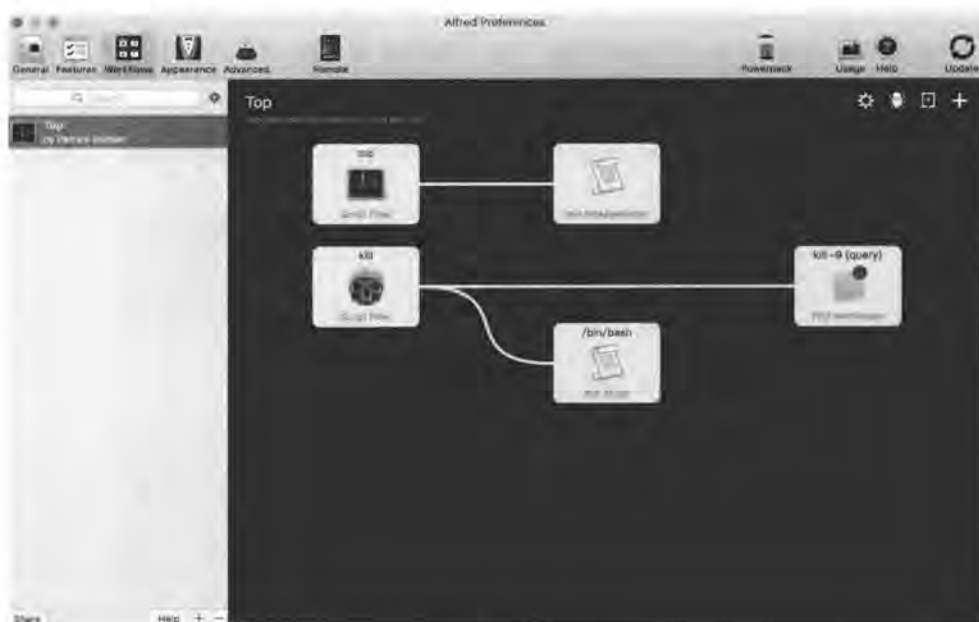
图 1.21 Alfred2 Workflows
