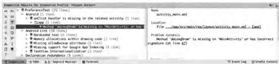
图 3.85 Inspect code
