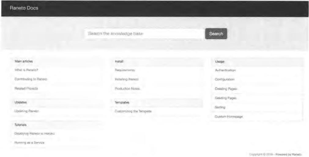
图 1.65 Raneto
