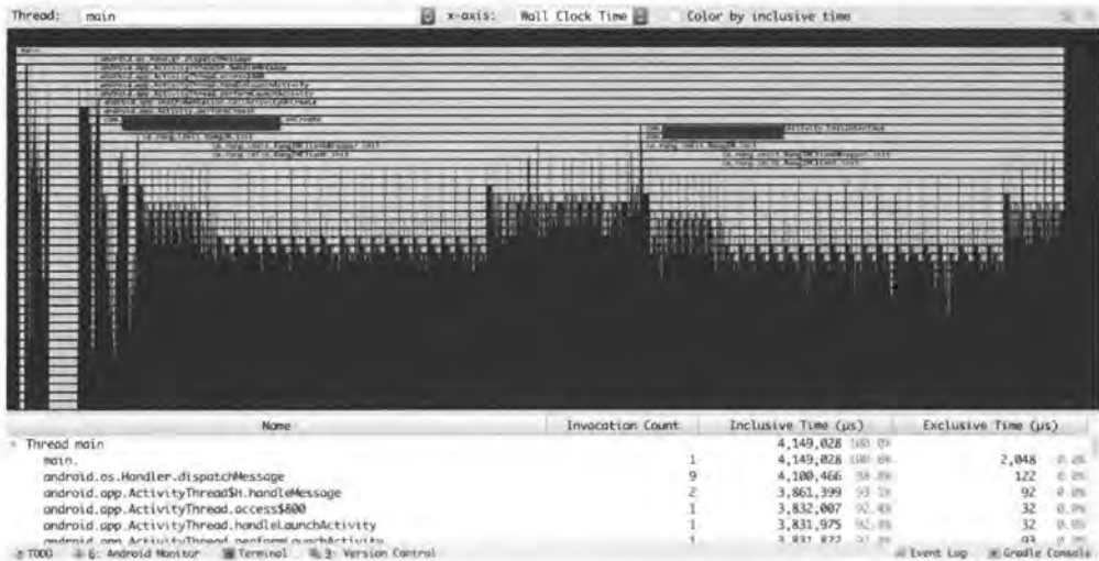
图 6.88 Method Tracing 数据
