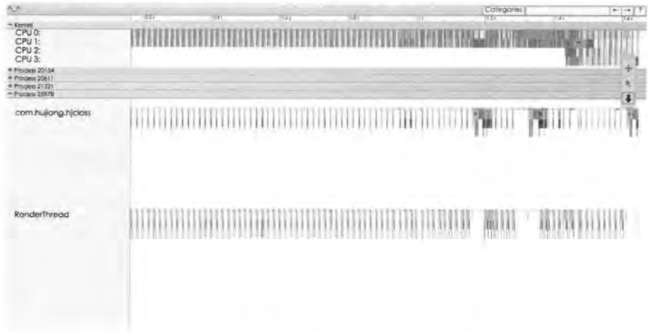
图 6.24 r21 版本 Systrace 数据结果图
