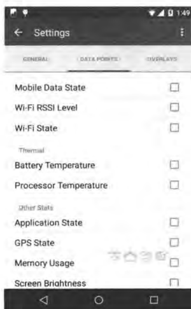
图 6.101 Trepn Profiler 性能数据
