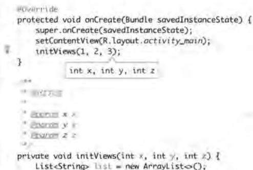
图 3.19 查看参数
