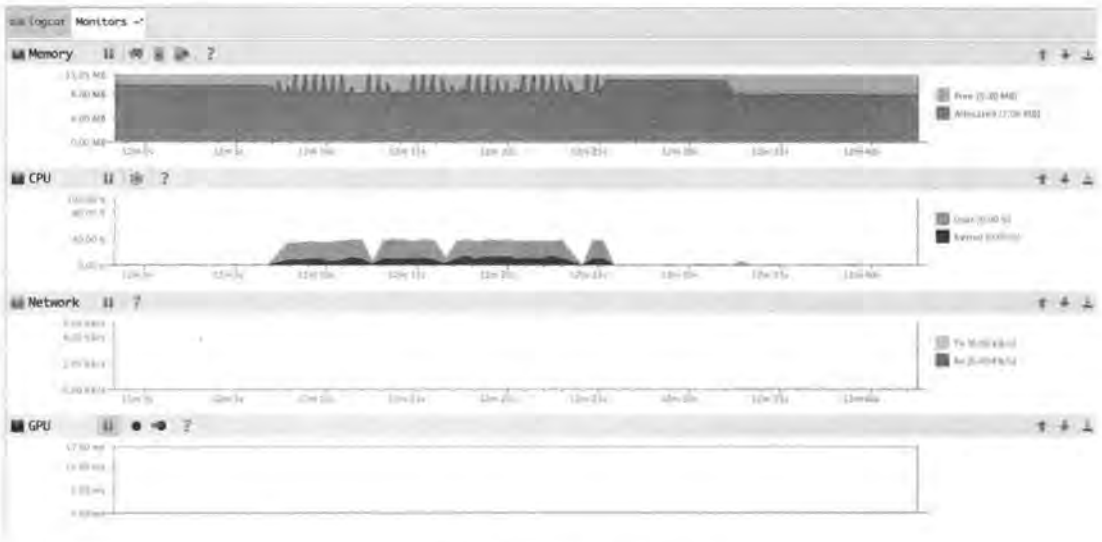
图 6.62 Memory Monitor
