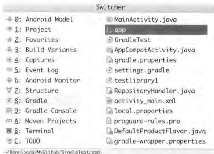
图 3.17 窗口导航
