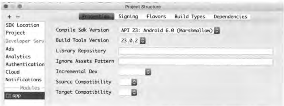
图 4.50 Project Structure
