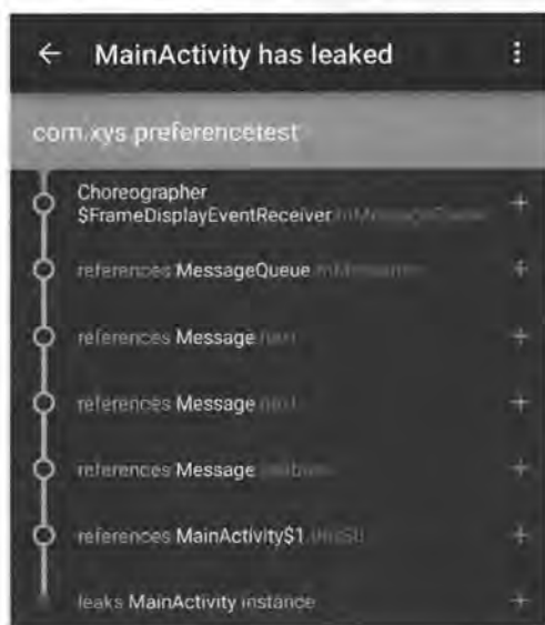
图 6.84 LeakCanary 信息
