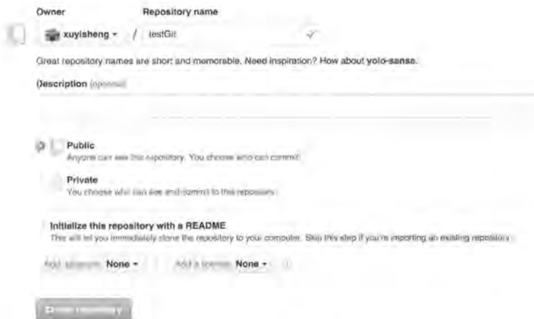
图 2.10 Repo 信息
