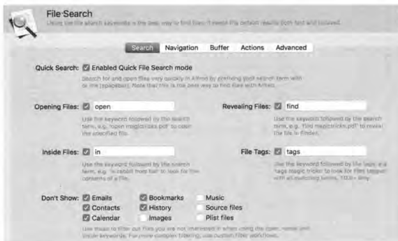
图 1.14 Alfred2 检索
