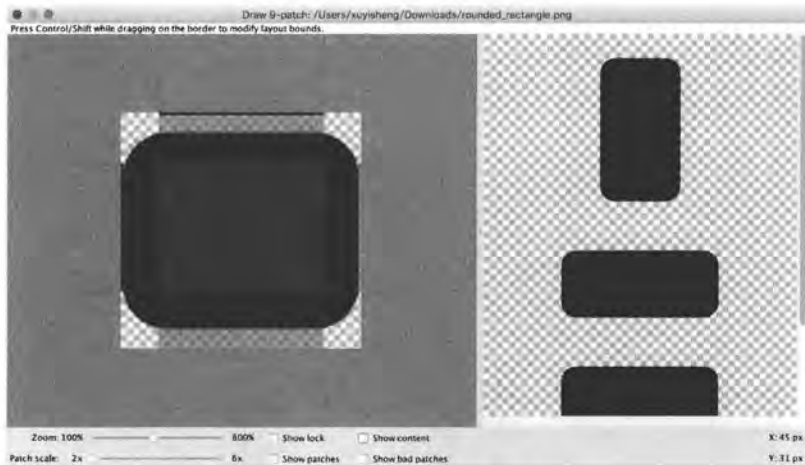
图 5.15 制作 9patch 图
