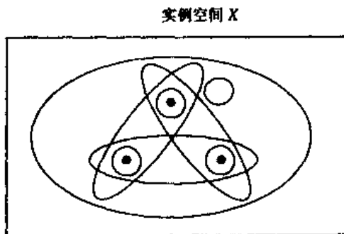
图 7-3 被 8 个假设拆散的包含 3 实例的集合
