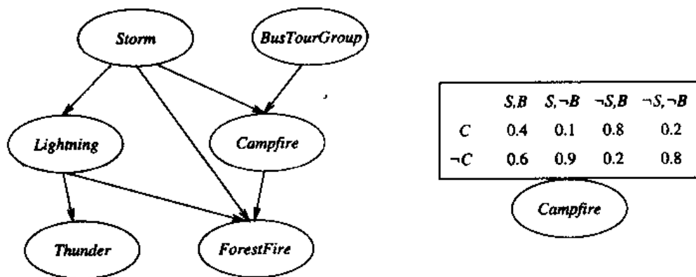
左边的网络表示了一组条件独立性假定。确切地说,每个节点在给定其父结点时,条件独立于其非后代结点。每个结点关联一个条件概率表,它指定了该变量在给定其父结点时的条件分布。右边列出了 Campfire 结点的条件概率表,其中 Campfire 、 Storm 和 BusTourGroup 分别缩写为 C, S, B
