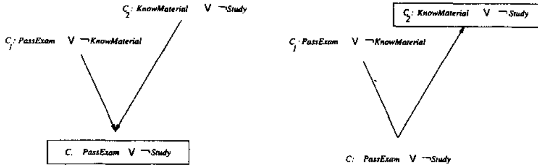
左边为应用归纳规则(演绎的)从给定子句 C_1 和 C_2 中推理出子句 C 。右边为其逆过程的应用(归纳的), 从 C 和 C_1 中推论出 C_2 。
