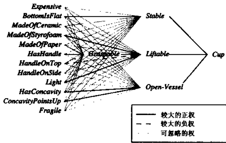
KBANN 使用训练样例来修改从领域理论中导出的网络权值。注意其中新产生的 Lifiable 对 MadeOfStyrofoam 和 HandleOnTop 的依赖性
