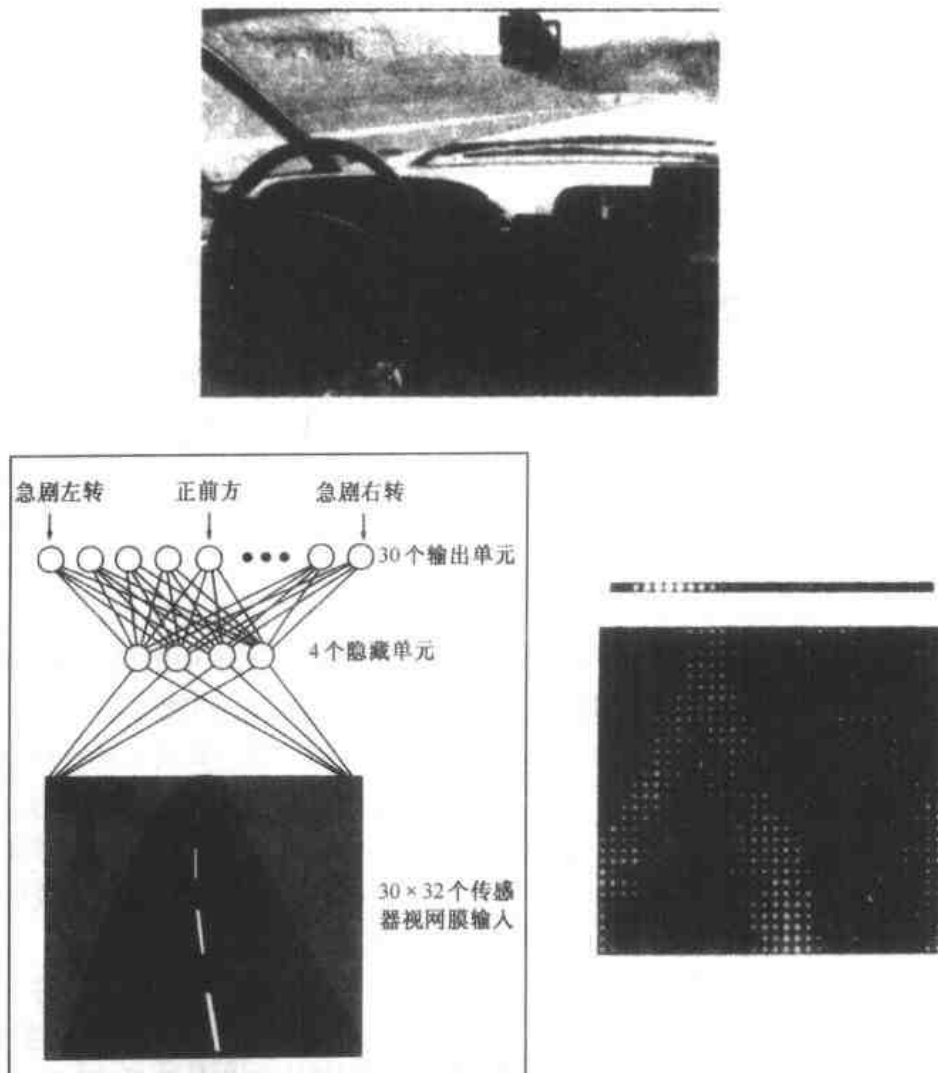
ALVINN 系统使用反向传播算法来学习驾驶汽车(上图),它的最高时速达到每小时 70 英里。左图显示了来自车前摄像机的图像是如何被映射到 960 个神经网络输入的,这些输入又前馈到 4 个隐藏单元,再连接到 30 个输出单元。网络输出编码了推荐的驾驶方向。右图显示了网络中一个隐藏单元的权值。进入这个隐藏单元的 30 \times 32 个权值显示在大的矩阵中,白色的方框表示正值而黑色的方框表示负权值。从这个隐藏单元到 30 个输出单元的权值被画在这个大矩阵上方的较小矩形中。从这些输出权值可以看出,激活这个隐藏单元会促使车向左转。
