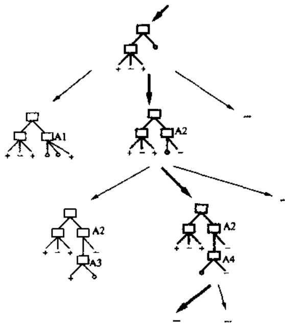
图 3-5 ID3 遍历可能决策树的空间,从最简单的树到逐渐复杂的树,其搜索由信息增益启发式规则引导
