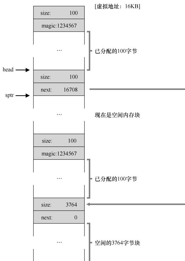
图 17.6 空闲空间和两个已分配的块
