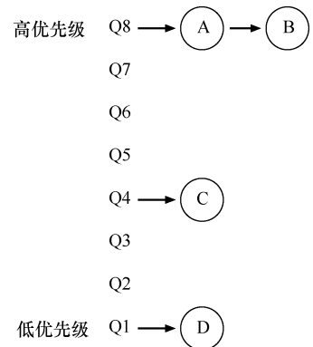
图 8.1 MLFQ 的例子
