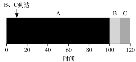
图 7.4 B 和 C 晚到时的 SJF
