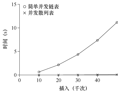
图 29.10 扩展散列表
