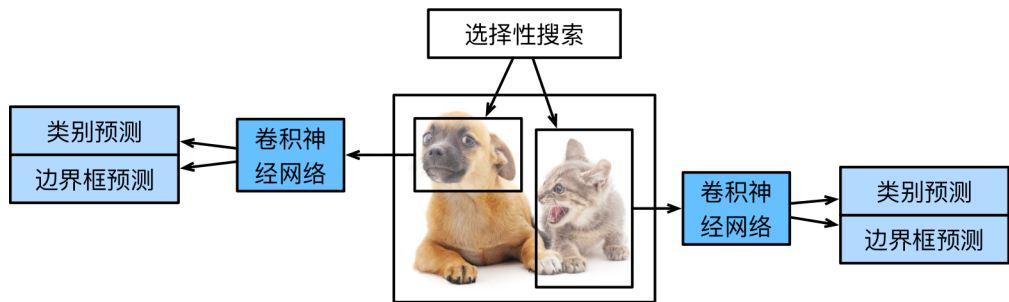
图 9.5: R-CNN模型
