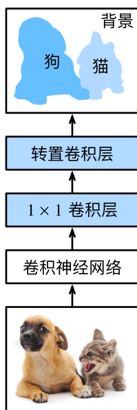
图 9.11: 全卷积网络
