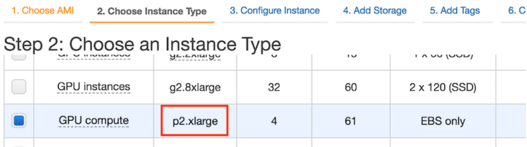
图 11.11: 选择实例
