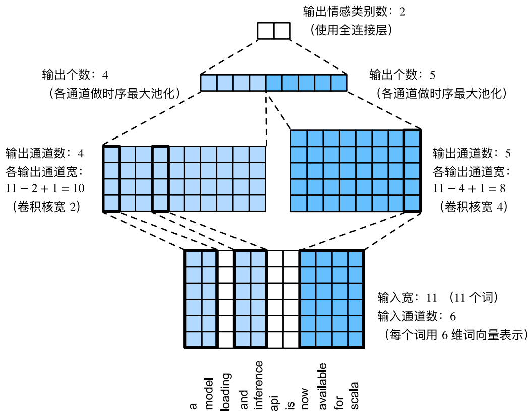
图 10.7: textCNN的设计
