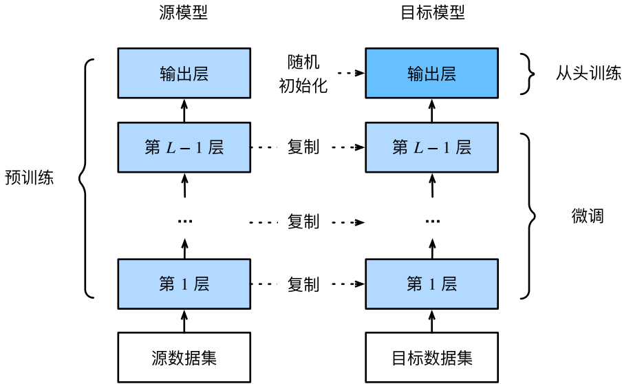
图 9.1: 微调
