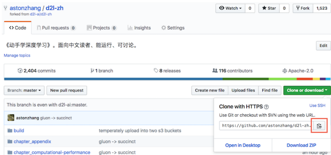
图 11.21: 复制代码库
