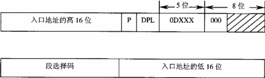
图 3.5 中断门和陷阱门的格式定义
