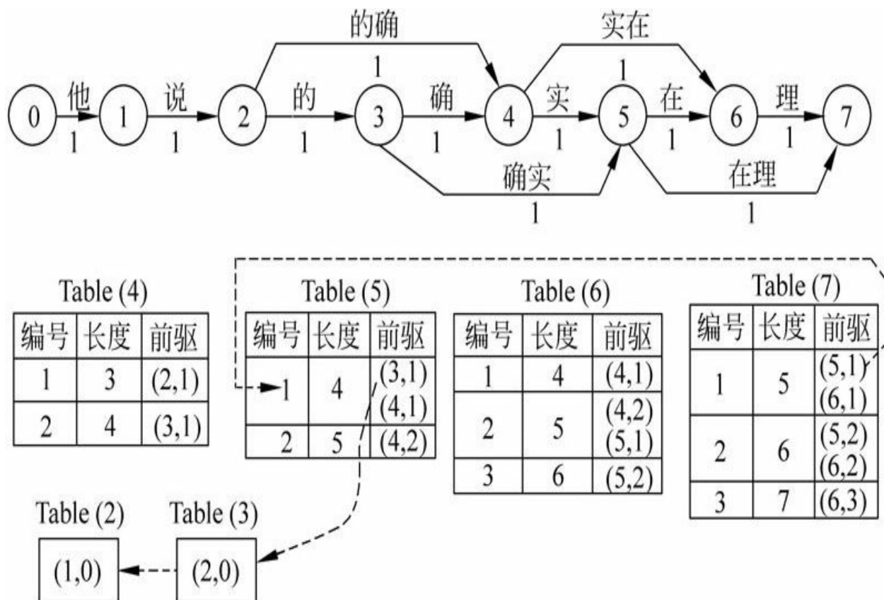
图7-2 句子“他说的确实在理”的求解过程 (N=3)
