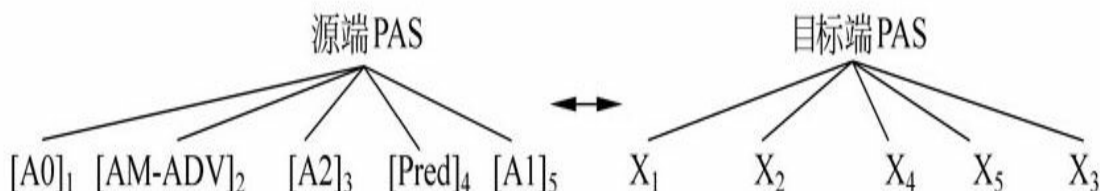
(b) 一条PAS转换规则
