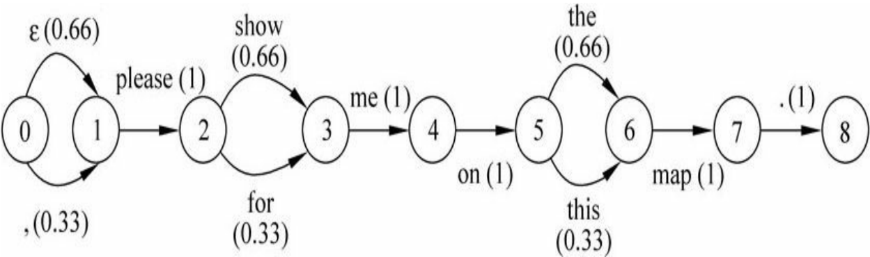
图11-34 混淆网络示例
