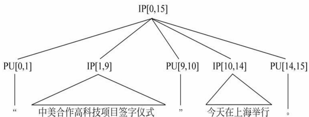
(b) 基本的 PCFG 模型在依存结构引导下生成的句法树
