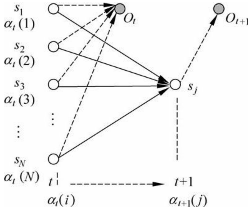
图6-7 前向变量的归纳关系
