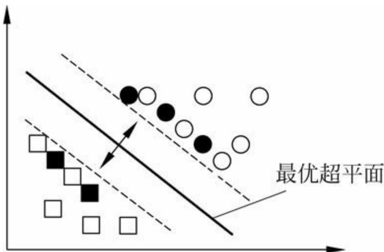
图2-6 最优超平面
