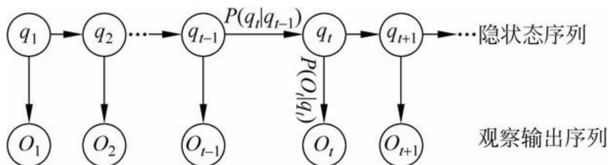
图6-5 HMM图解
