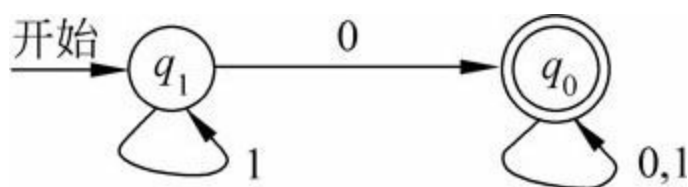
图3-5 DFA例子
