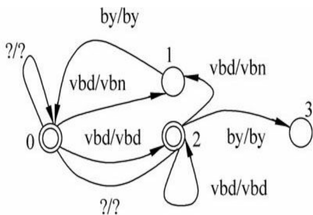
(b) T_2 的局部扩展
