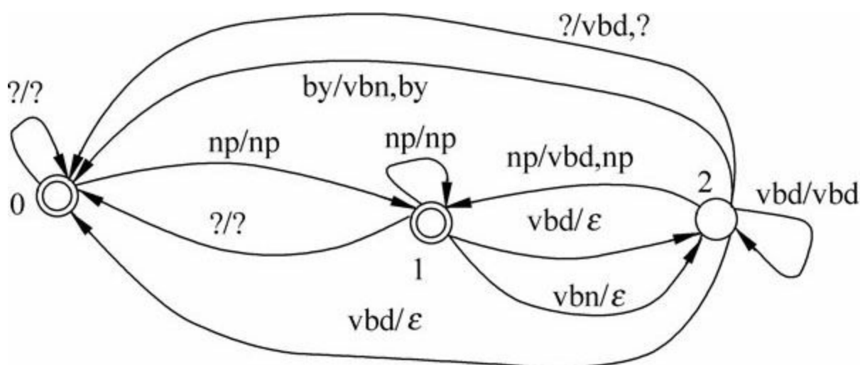
图3-15 确定性的 T_3
