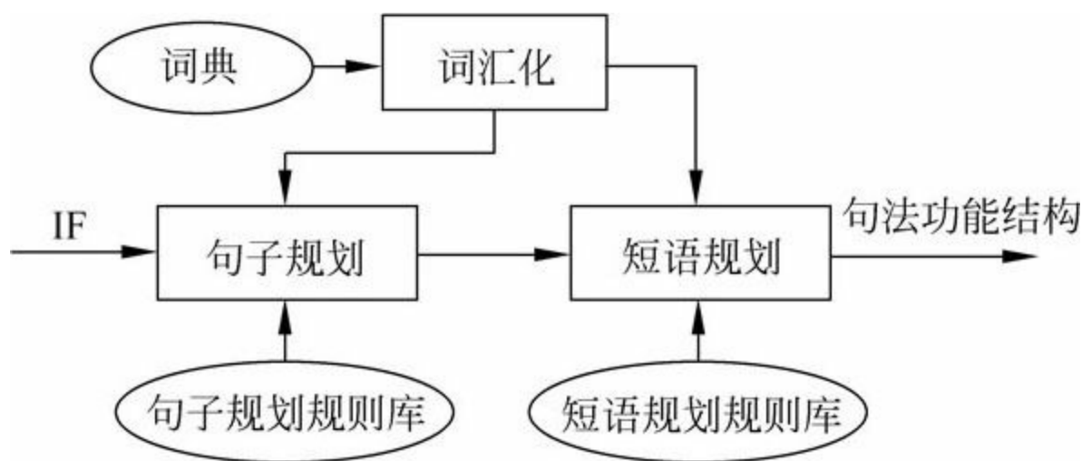
图16-8 微观规划器结构图
