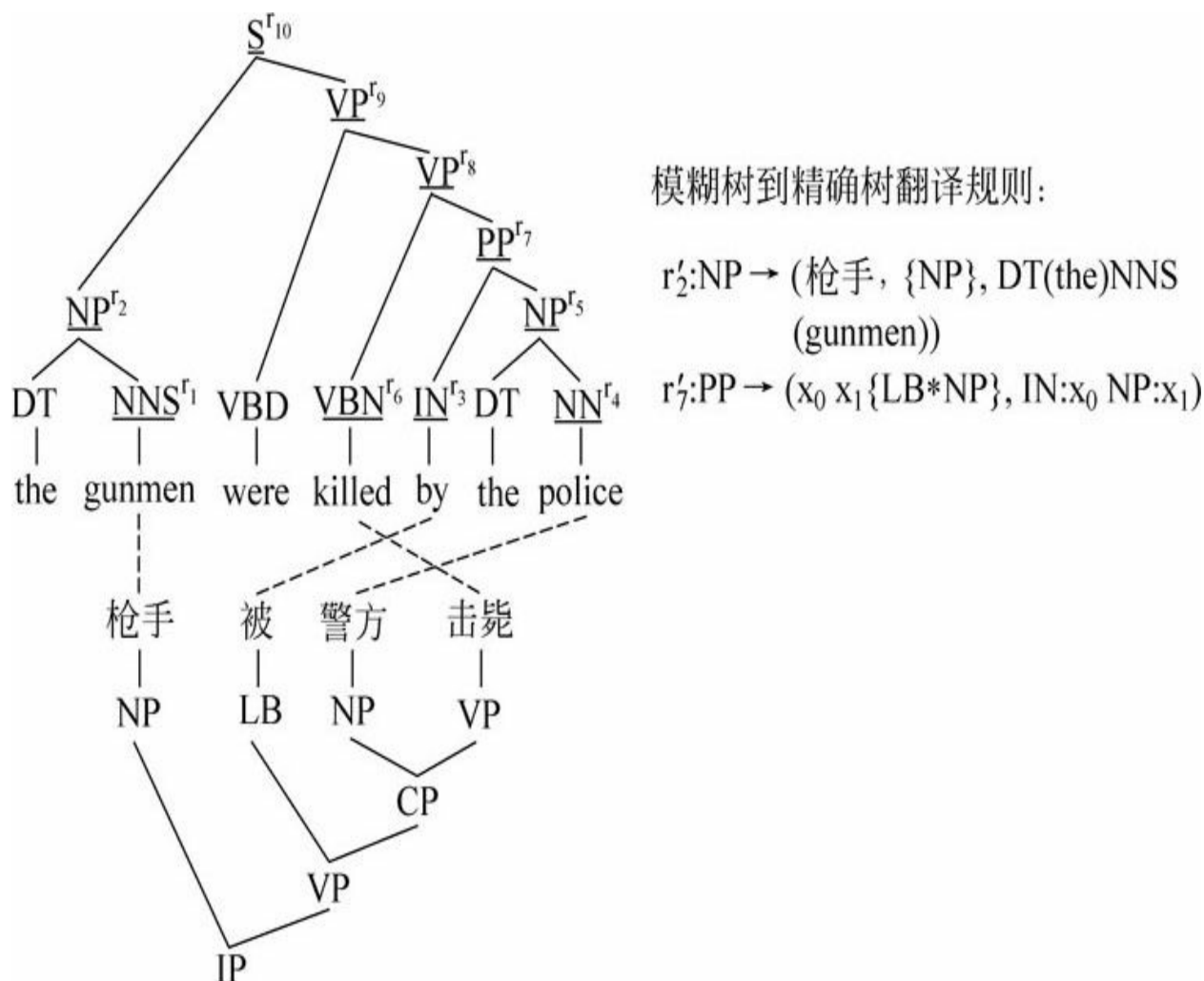
图11-24 模糊树到精确数翻译规则抽取示例
