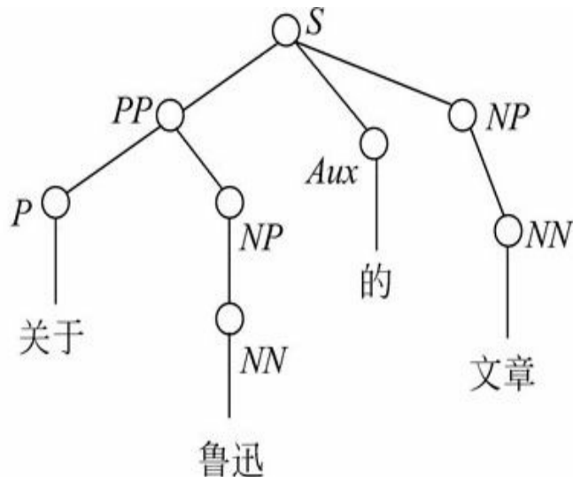
(b) CFG 的派生树示例2
