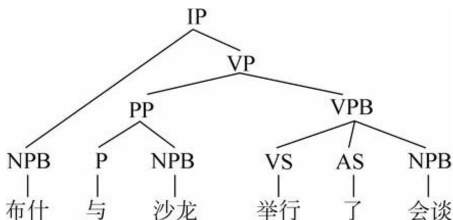
图11-20 对应中文句子“布什与沙龙举行了会谈”的一棵句法树
