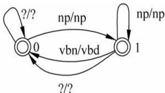
(b) T_1 的局部扩展
