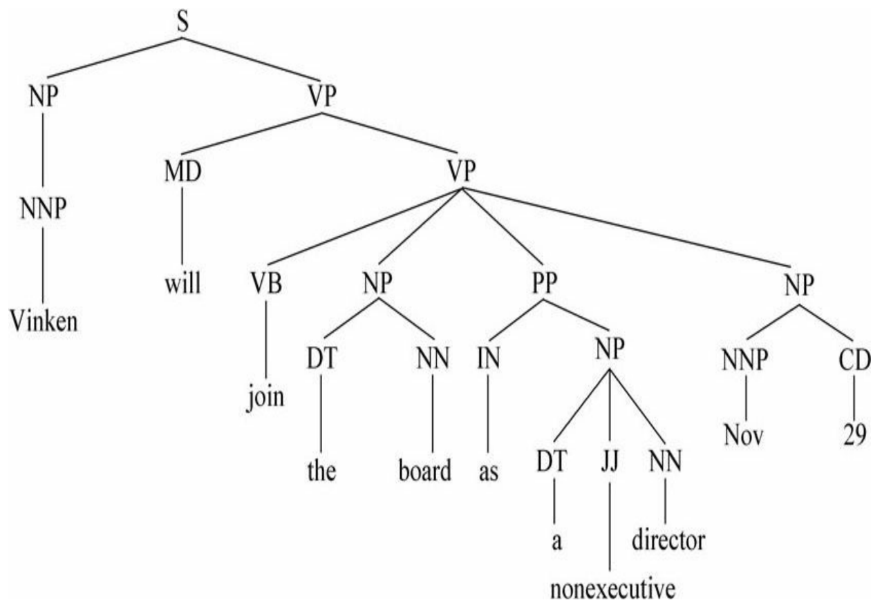
图8-27 短语结构分析树
