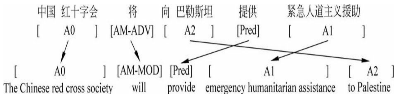
(a) 一个双语联合语义角色标注的例子
