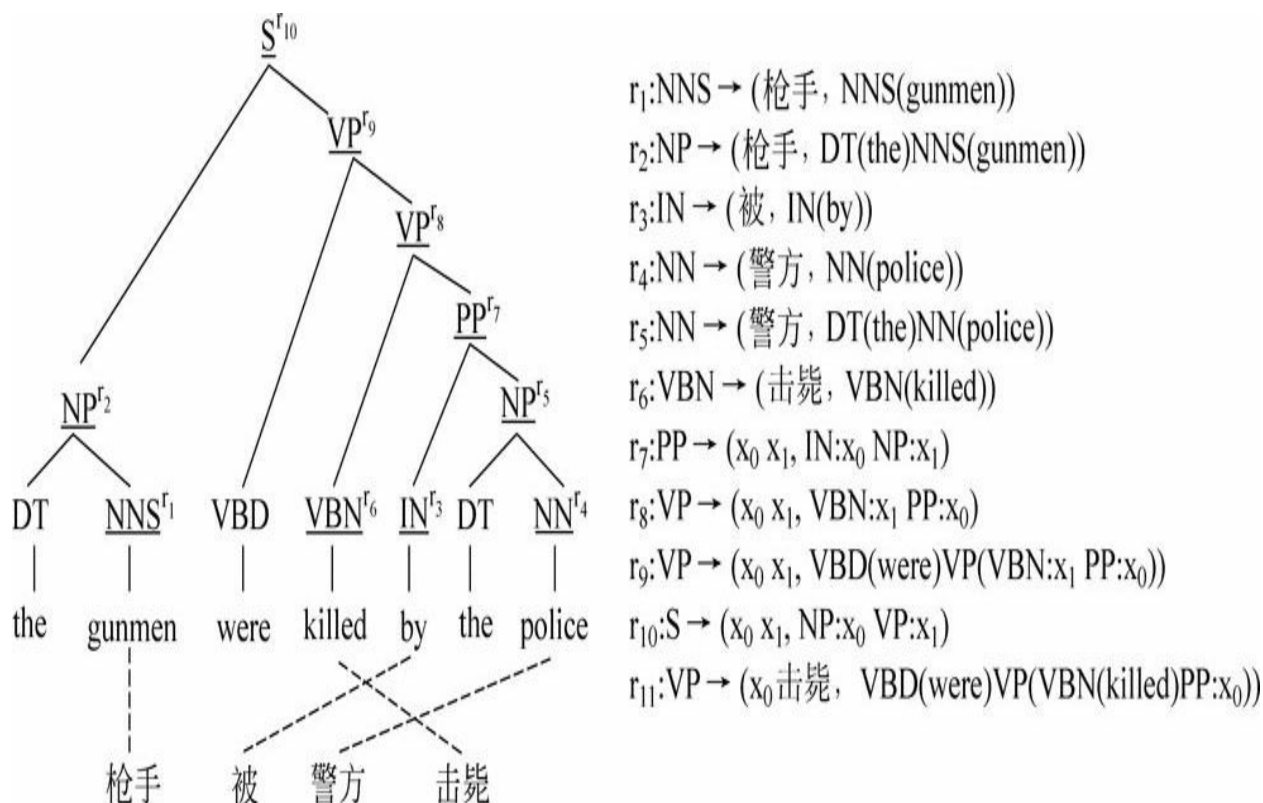
图11-22 同步树替换规则抽取实例
