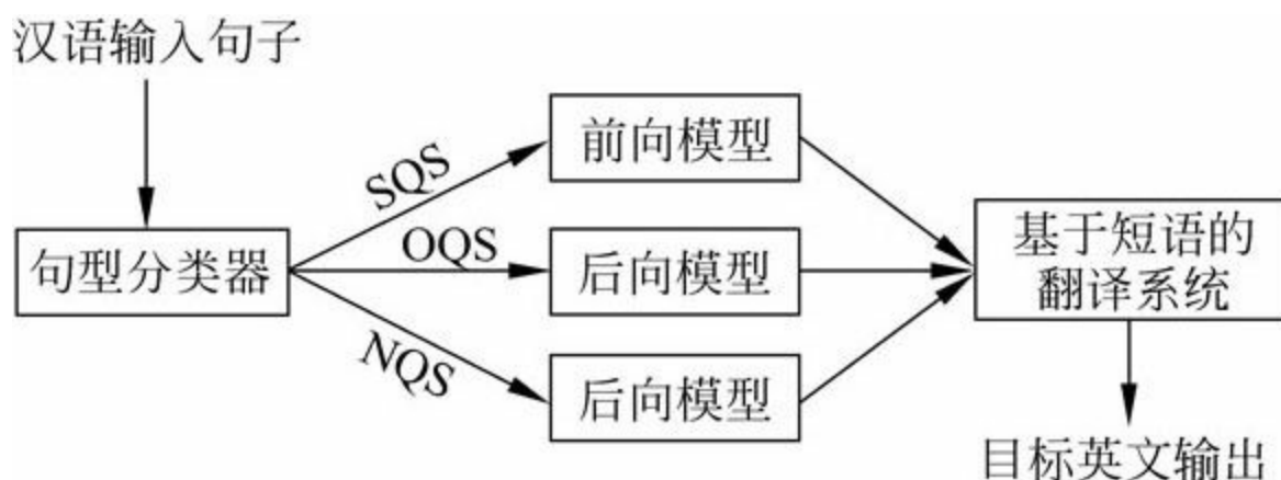
图12-9 基于源语言句型的翻译框架
