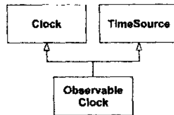
图 24.8 用 C++ 的多重继承分离 Clock 和 TimeSource
