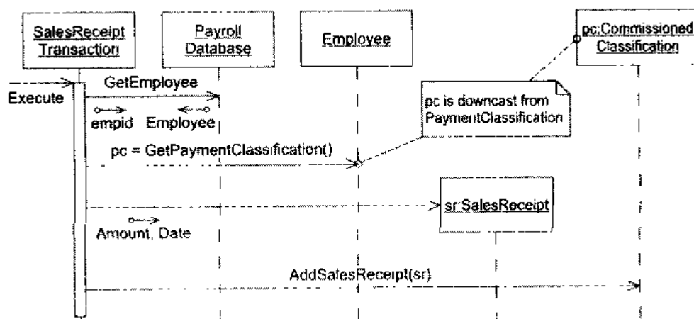
图 19.10 SalesReceiptTransaction 的动态模型
