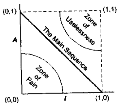
图 20.13 被排除的区域
