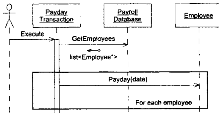
图 19.30 PaydayTransaction 动态模型
