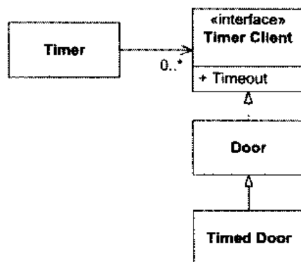
图 12.1 位于层次结构顶部的 Timer Client
