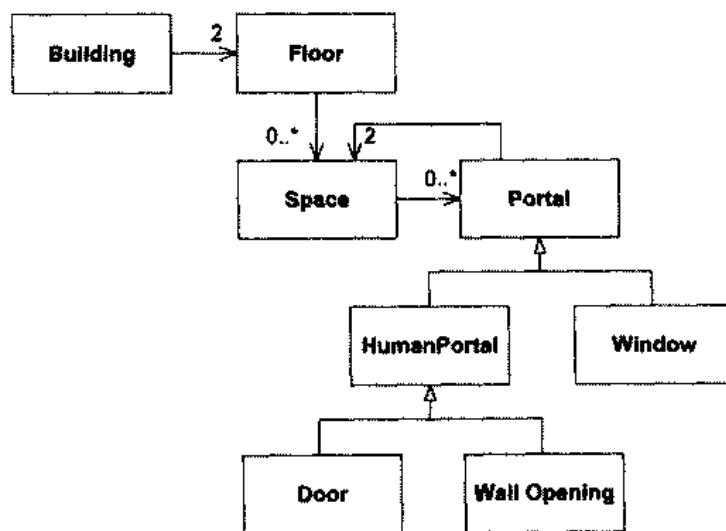
图 30.4 楼层平面数据结构
