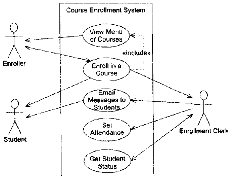
图 A.1 系统边界图
