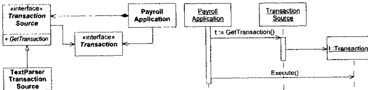
图 19.35 主程序的动态模型
