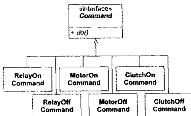
图 13.2 复印机软件中一些简单的 Command
