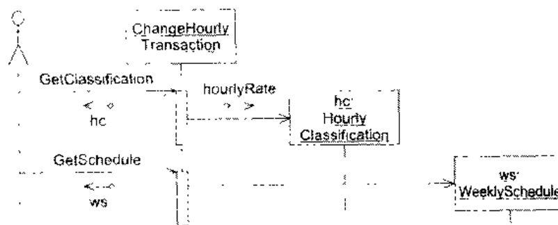
图 19.19 ChangeHourlyTransaction 的动态模型
