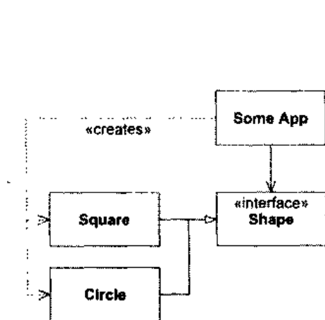
图 21.1 违反 DIP 原则创建具体类的应用程序
