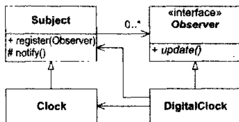
图 24.12 拉模型 OBSERVER 模式的规范形式
