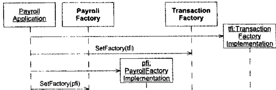
图 22.10 主程序和对象工厂的动态结构
