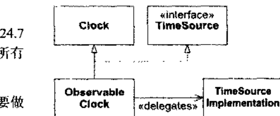
图 24.10 ObservableClock 的委托方法实现
