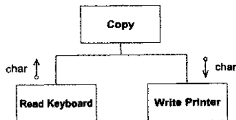
图 7.1 Copy 程序结构图
