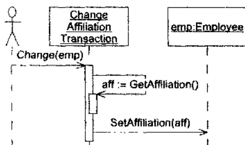
图 19.26 ChangeAffiliationTransaction 动态模型
