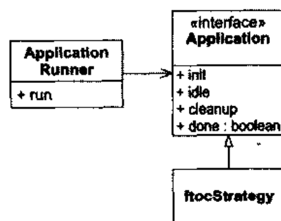
图 14.2 Application 算法策略
