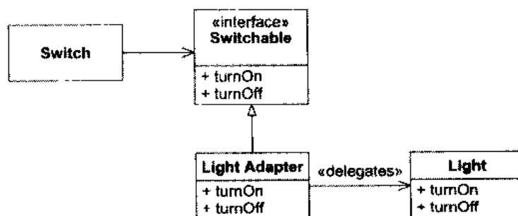
图 25.4 使用 ADAPTER 模式解决台灯问题
