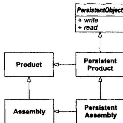
图 26.9 STAIRWAY TO HEAVEN 模式
