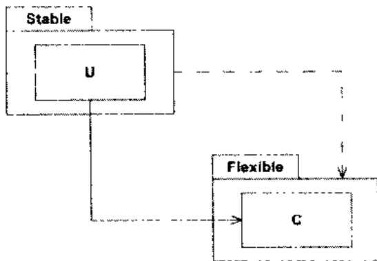
图 20.10 糟糕依赖关系的原因
