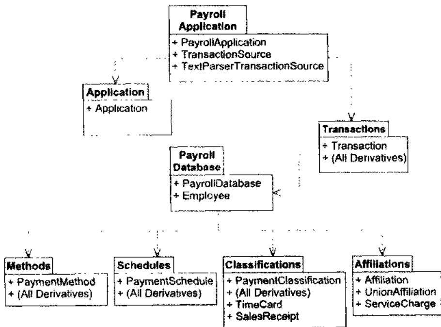
图 22.1 可能的薪水支付应用程序包图
