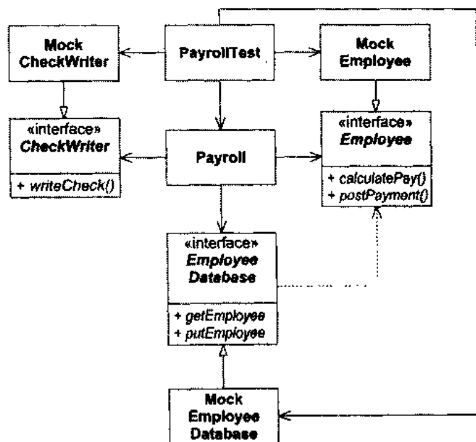
图 4.2 使用 Mock Objects 测试方法，解除了耦合的薪水支付应用模型
