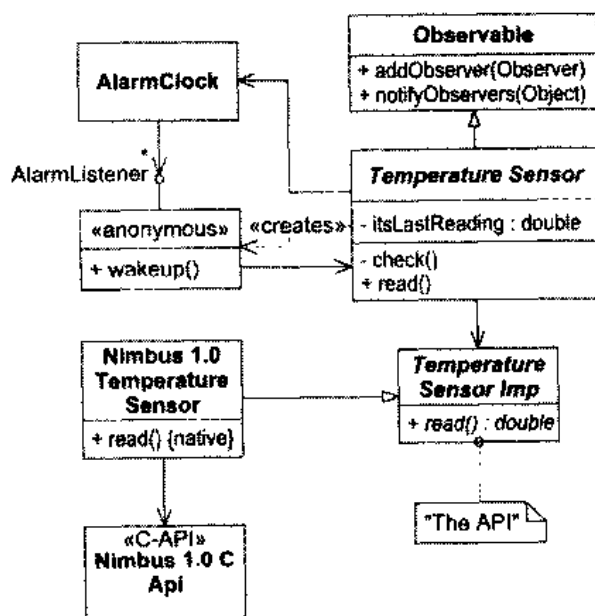
图 27.9 具有 API 的温度传感器
