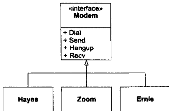
图 28.1 Modem 层次结构
