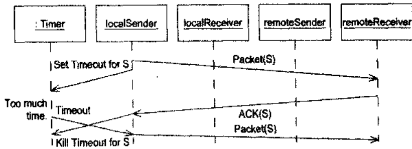
图 B.12 ACK/重传竞争条件
