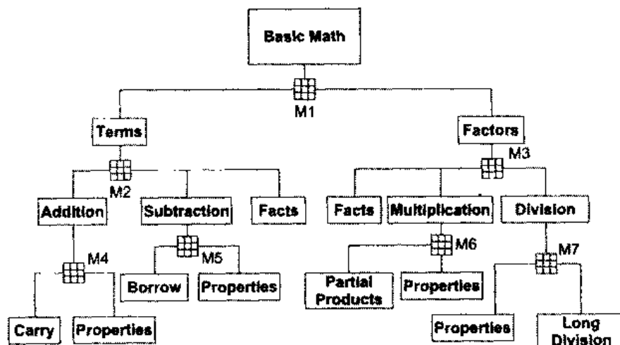
图 30.1 基础数学的考察点层次结构
