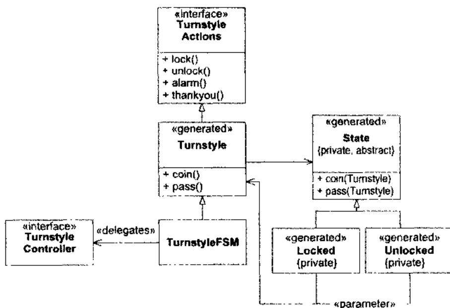
图 29.5 3 层 FSM
