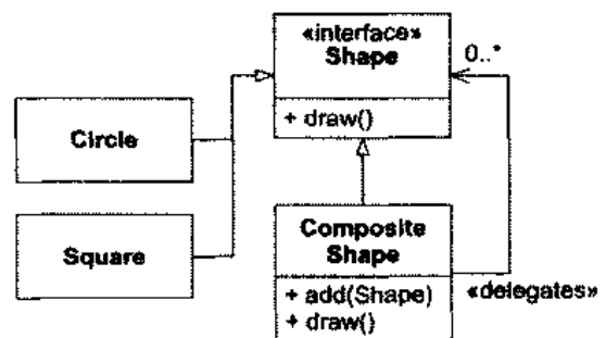
图 23.1 Composite 模式
