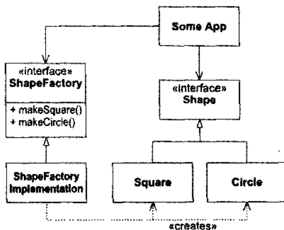
图 21.2 Shape 工厂
