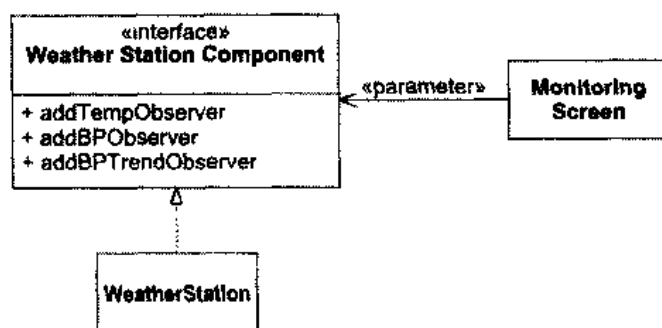
图 27.15 WeatherStation 抽象接口
