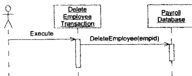
图 19.6 DeleteEmployee 操作的动态模型
