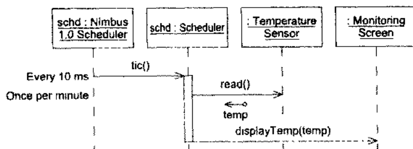
图 27.3 初始的调度器顺序图 (sequence diagram)
