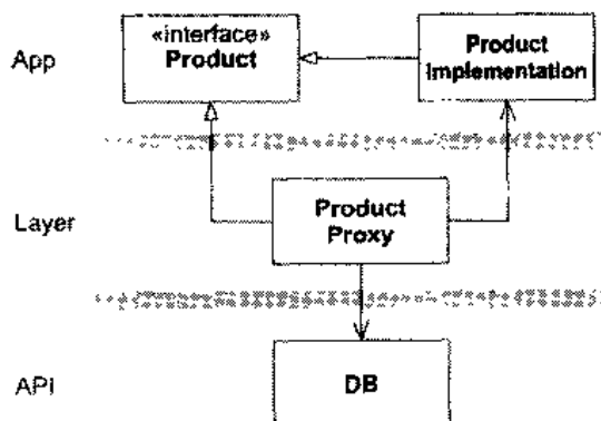
图 26.8 PROXY 模式是如何倒置应用程序和层之间的依赖关系的
