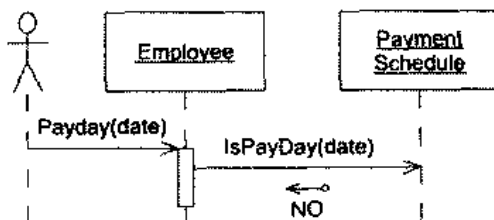
图 19.31 动态模型情景：“今天不是发薪日”
