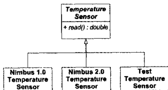
图 27.1 初始的温度传感器设计
