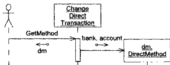
图 19.23 ChangeDirectTransaction 动态模型
