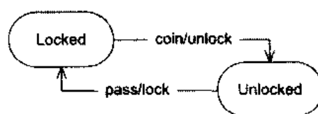
图 29.1 简单的十字转门状态机
