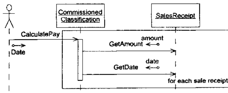
图 18.9 计算应支付佣金雇员的薪水
