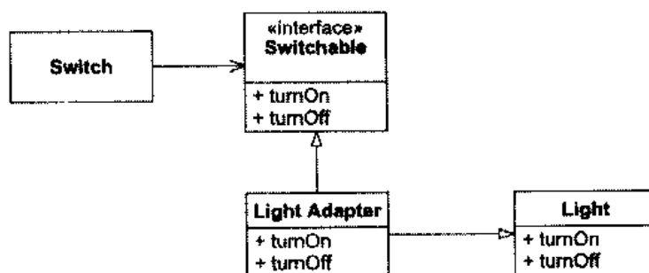
图 25.5 使用 ADAPTER 模式解决台灯问题
