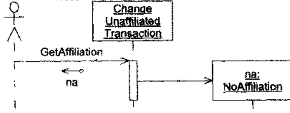
图 19.28 ChangeUnaffiliatedTransaction 动态模型
