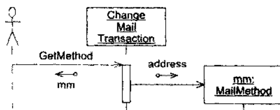
图 19.24 ChangeMailTransaction 动态模型
