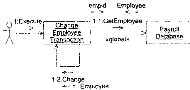
图 19.15 ChangeEmployeeTransaction 的动态模型
