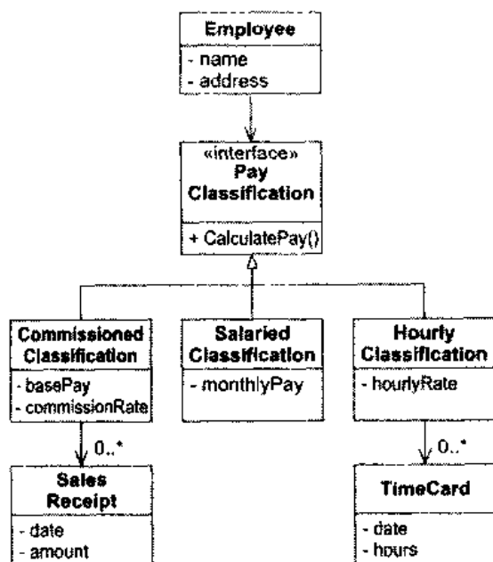
图 13.4 雇员数据库
