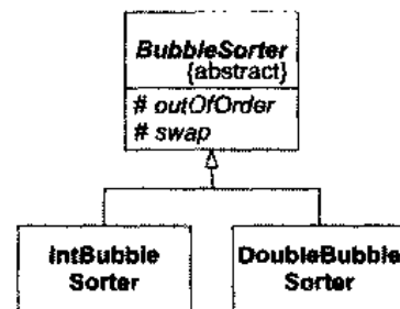
图 14.1 Bubble-Sorter 结构
