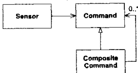
图 23.3 组合命令
