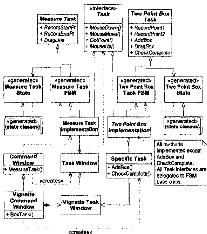
图 30.13 Taskmaster 构架
