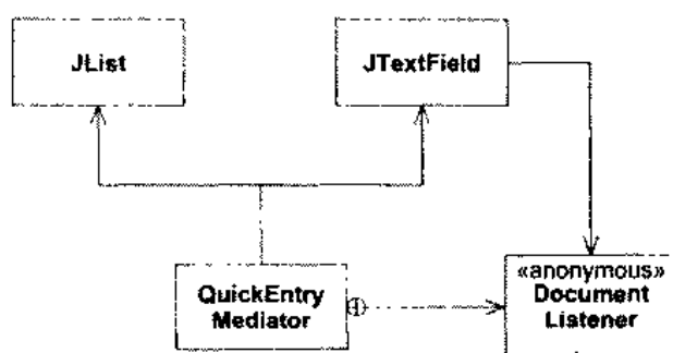
图 15.2 QuickEntryMediator
