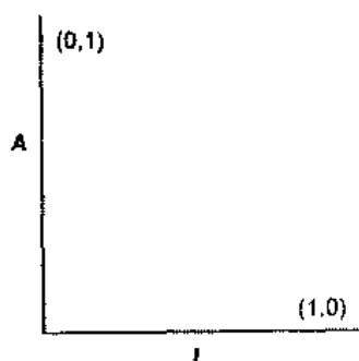
图 20.12 A-I 坐标图
