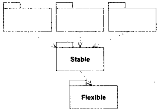
图 20.9 违反了 SDP
