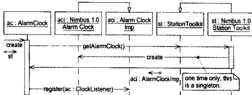
图 27.12 创建 AlarmClock
