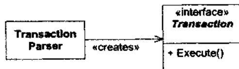
图 19.1 Transaction 接口
