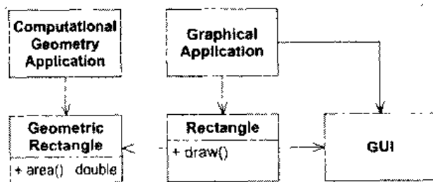
图 8.2 分离的职责
