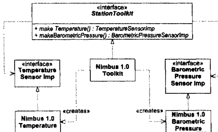
图 27.10 StationToolkit
