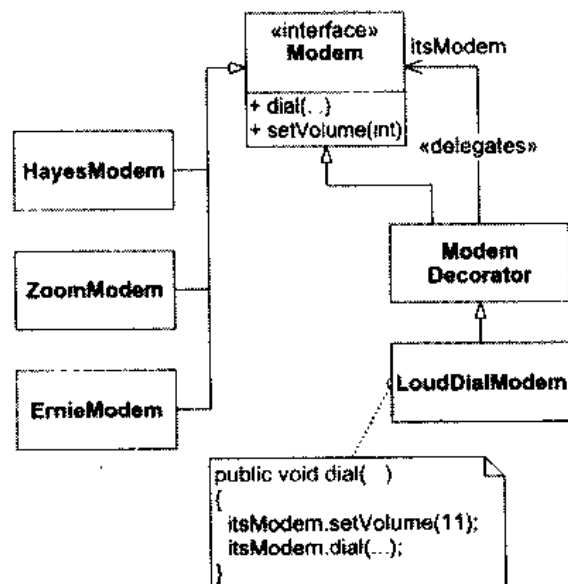
图 28.6 ModemDecorator
