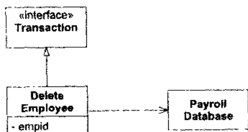
图 19.5 DeleteEmployee 操作的静态模型
