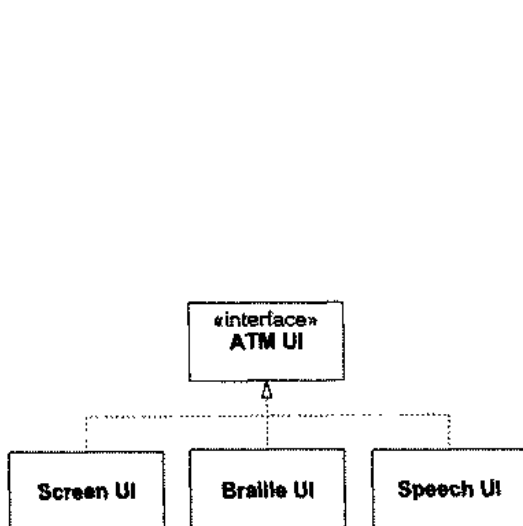
图 12.4 ATM 界面层次结构
