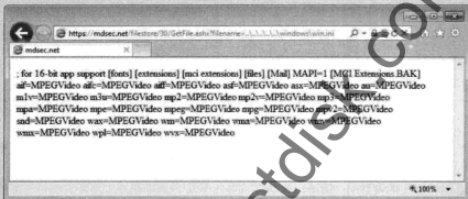
图10-5 成功的路径遍历攻击
