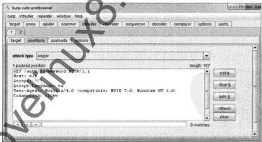
图4-7 使用Burp Intruder对部分文件名实施定制蛮力攻击
