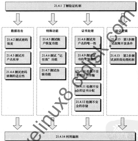
图21-5 测试验证机制
