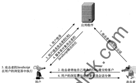
图12-3 反射型XSS攻击的实施步骤
