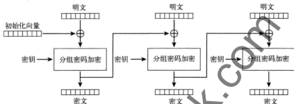
图7-5 使用CBC密码时，在加密每个明文分组之前，将它与上一个密文分组进行XOR运算
