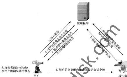
图12-4 保存型XSS漏洞的实施步骤
