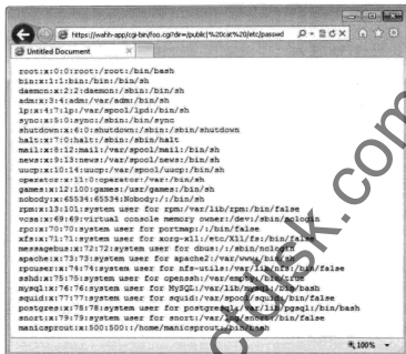
图10-2 一个成功的命令注入攻击
