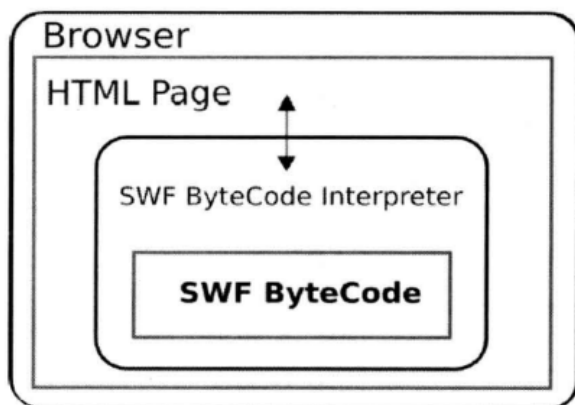
▲图 6-3 浏览器解释 SWF 的过程
