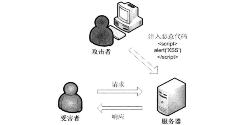
▲图 1-17 持久型 XSS 攻击流程
