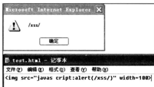
▲图 1-32 利用 Tab 拆分关键字
