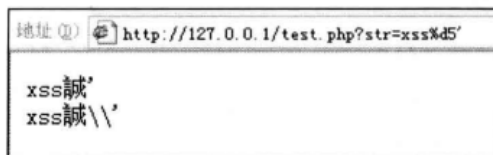
▲图 7-58 注入非法字符集序
