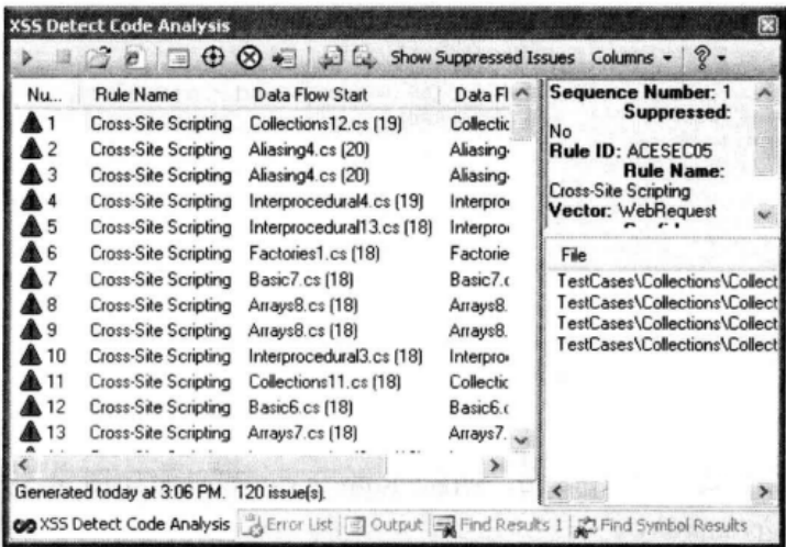
▲图 4-2 XSSDetect 界面
