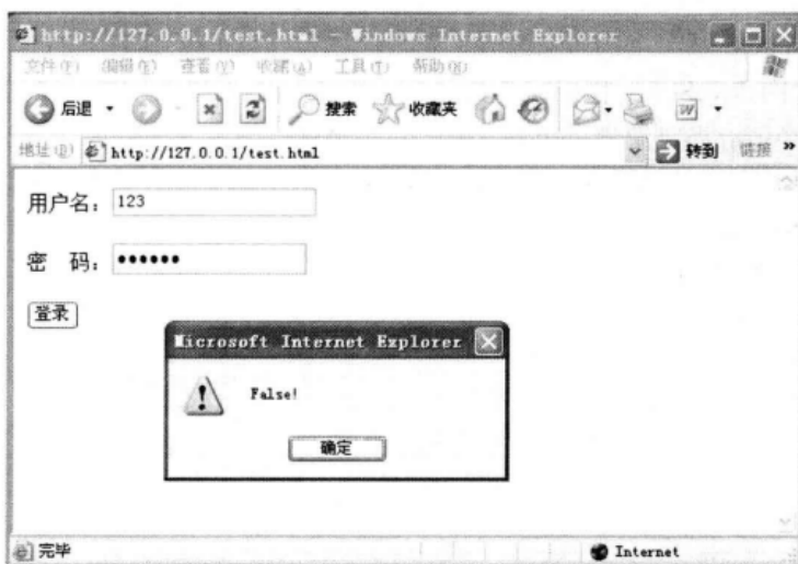
▲图 5-10 提示错误
