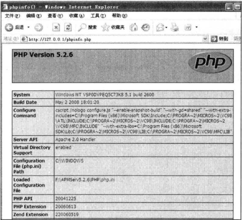
▲图 4-26 Phpinfo 页面
