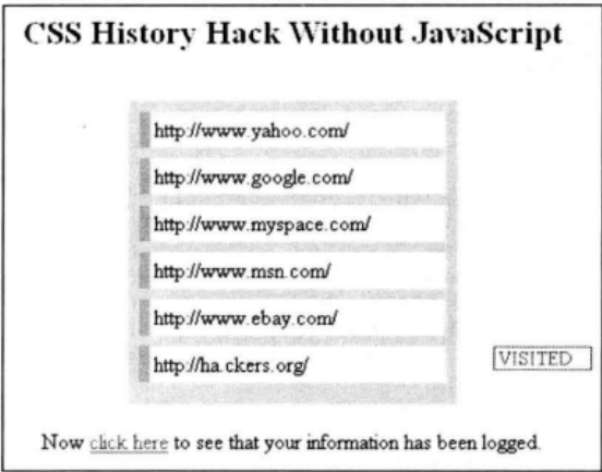
图 2-27 Rsnake 的 POC
