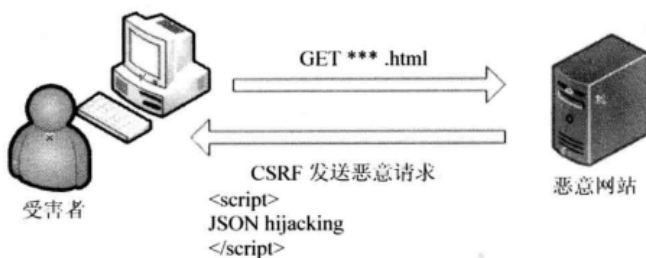
▲图 7-11 步骤②
