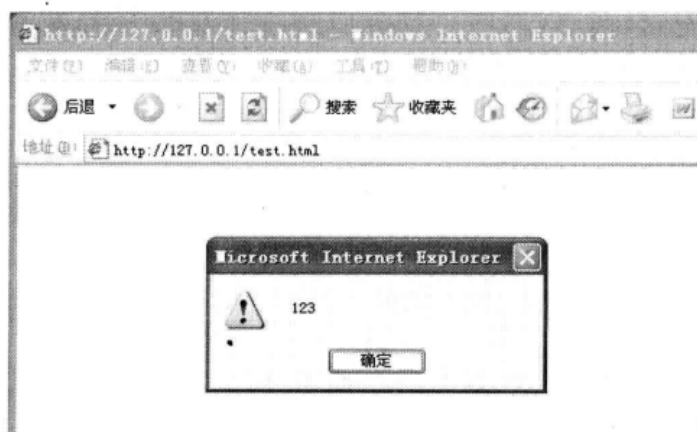
▲图 6-18 执行 XSS
