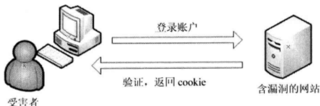
▲图 7-10 步骤①
