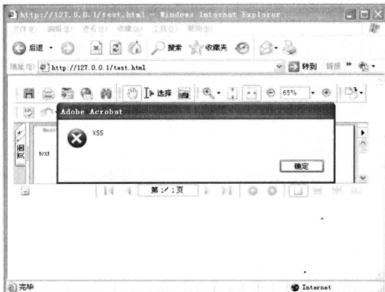
▲图 7-36 触发 XSS
