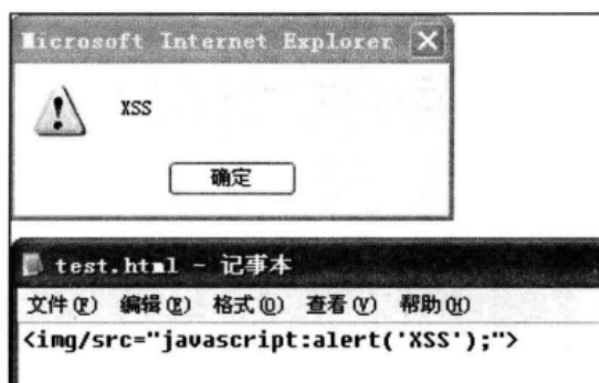
▲图 1-40 插入/字符
