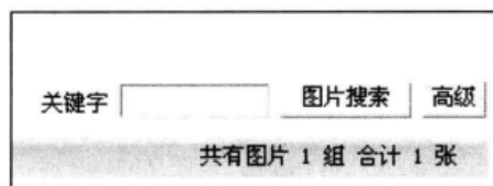
▲图 2-4 搜索模块
