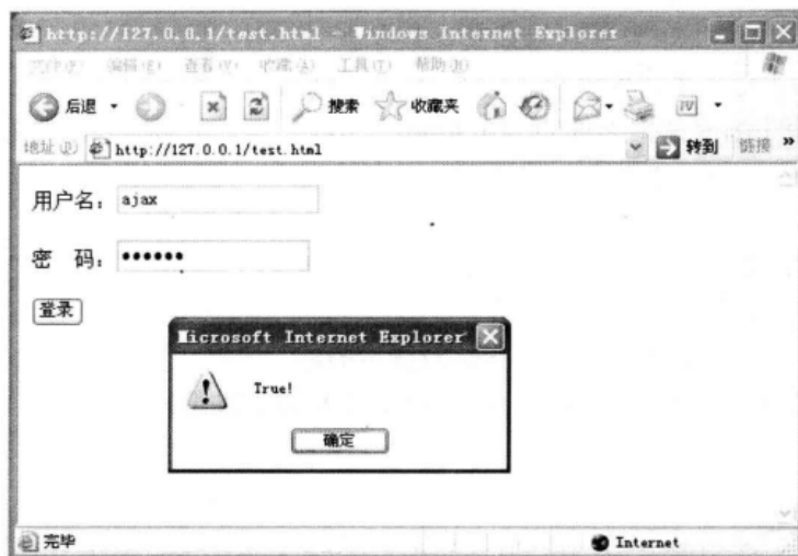
▲图 5-9 提示正确
