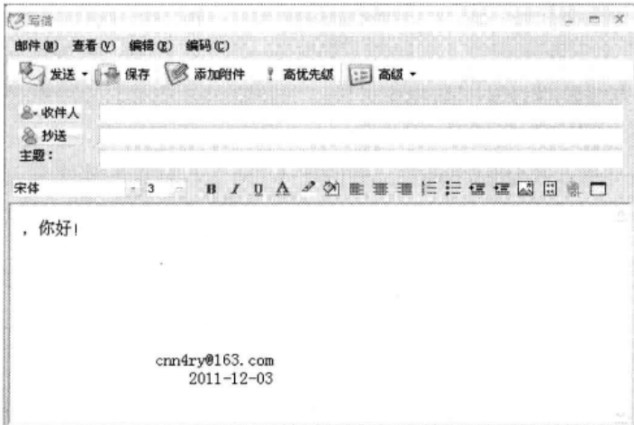
▲图 7-43 写信窗口
