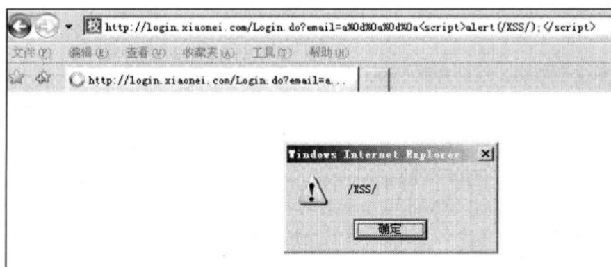
▲图 7-15 触发 HRS/XSS
