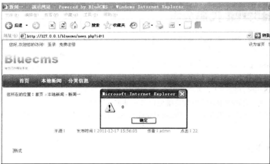
▲图 4-13 执行 XSS
