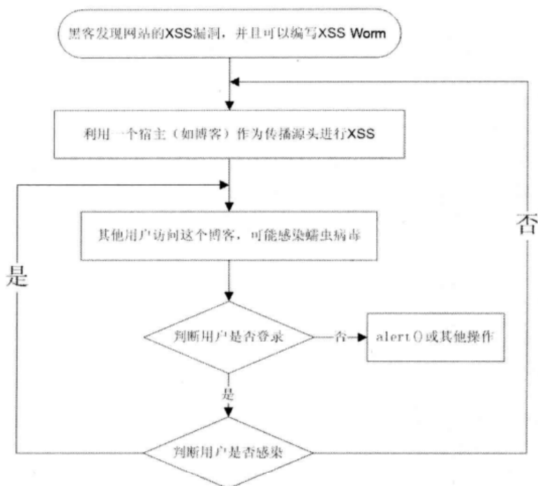
▲图 5-13 XSS 蠕虫攻击过程示意图
