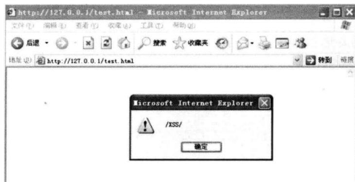
▲图 7-27 触发 XSS
