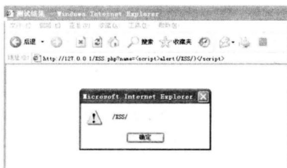
▲图 1-10 触发 XSS
