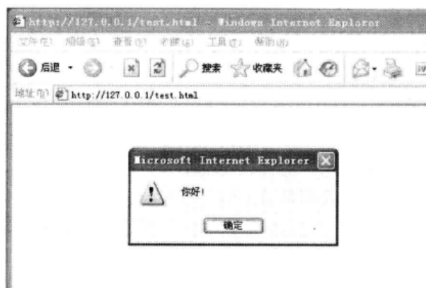
▲图 6-24 执行 XSS
