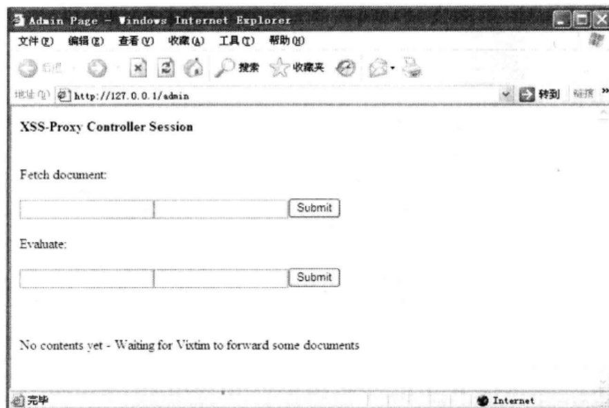
▲图 3-26 XSS-Proxy 界面
