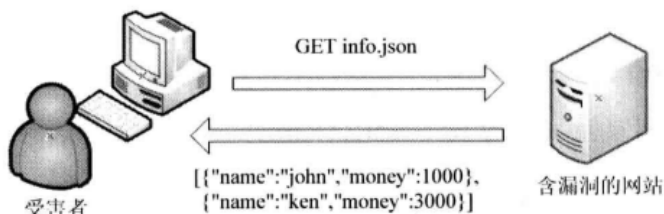
▲图 7-12 步骤③
