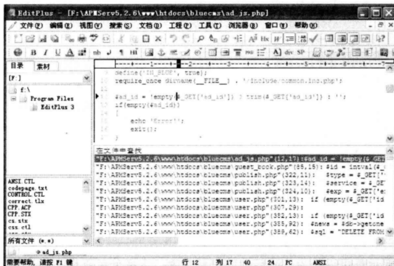
▲图 4-8 查找结果
