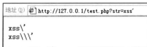
▲图 7-57 注入引号
