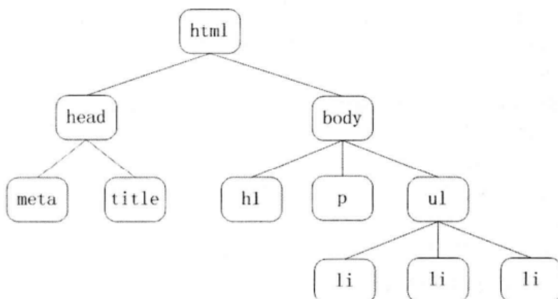
▲图 4-17 DOM 模型
