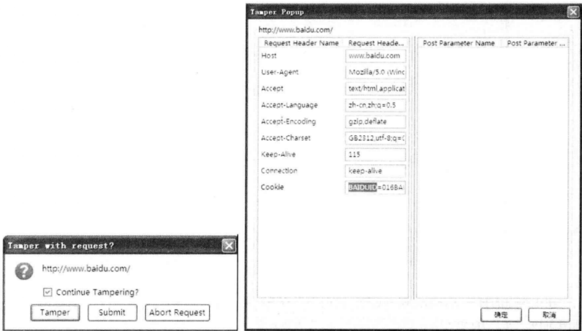
▲图 3-15 start tamper
