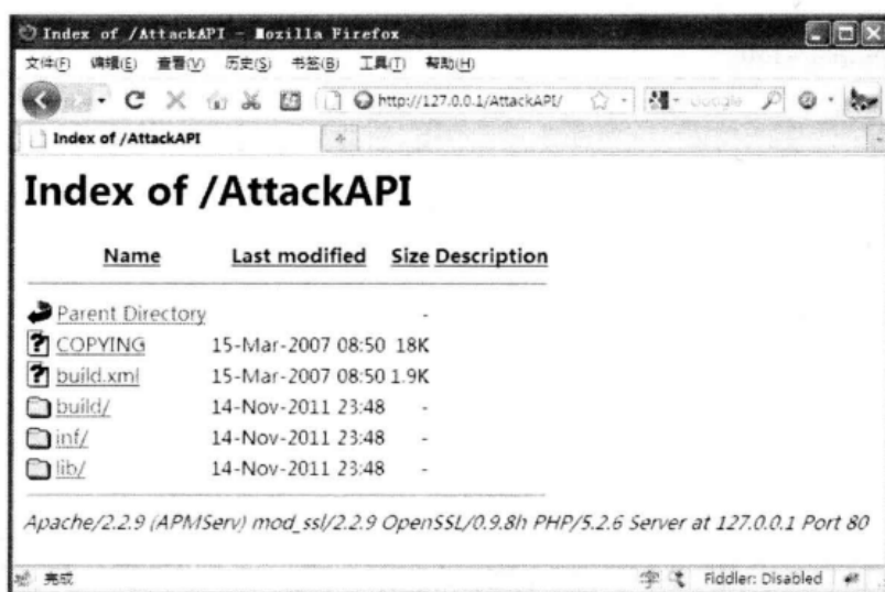
▲图 3-42 AttackAPI 界面
