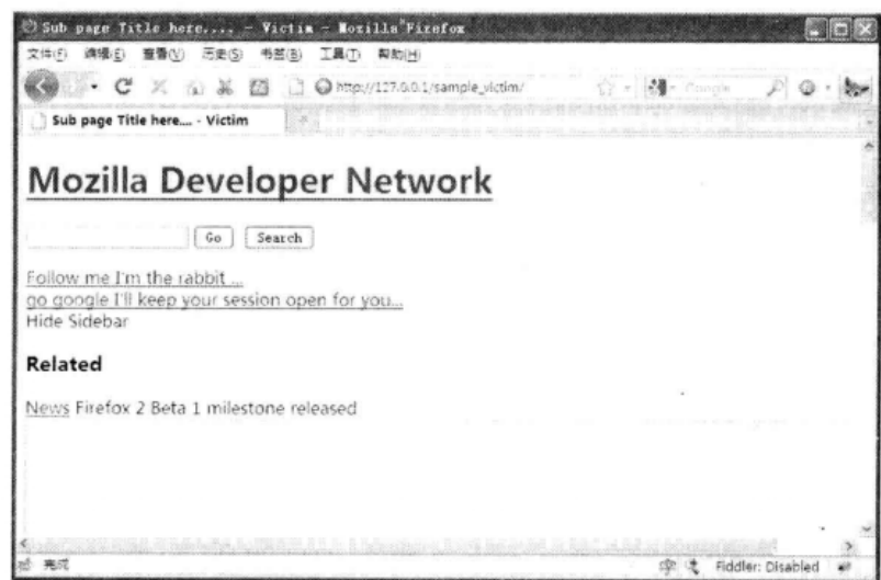
▲图 3-36 打开 Sample-Victim
