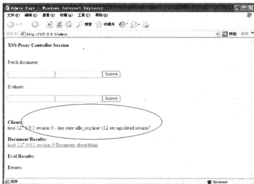
▲图 3-27 上线提示
