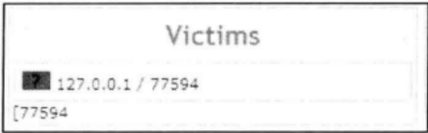
▲图 3-37 提示上线
